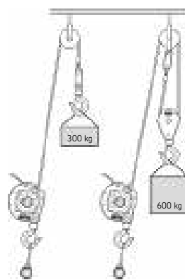
am Boden fixierter PULLEYMAN
