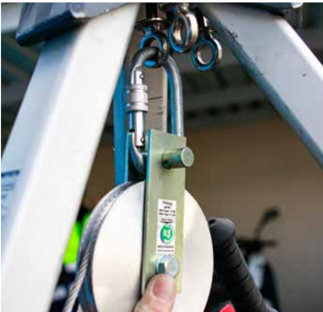
Abb. 39 + 40: Den Bolzen bis zum Anschlag durch die beiden Bohrungen an der Seilrolle stecken und die Beilagscheibe auflegen.
